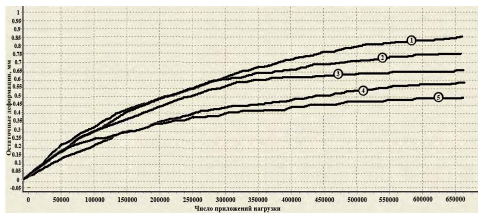
Рис. 3. Накопление остаточных деформаций в щебеночно-песчаных смесях, укрепленных комплексным вяжущим: 1 — ЩПС, укрепленная 3 % цемента + 5 % битумной эмульсии; 2 — ЩПС, укрепленная 3 % цемента + 3 % битумной эмульсии; 3 — ЩПС, укрепленная 5 % цемента + 3 % битумной эмульсии; 4 — ЩПС укрепленная 3 % цемента + 3 % битумной эмульсии + папоСТАВ; 5 — ЩПС, укрепленная 3 % цемента + 3 % битумной эмульсии + ANТ
